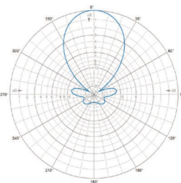
H-Plane | 405 MHz
