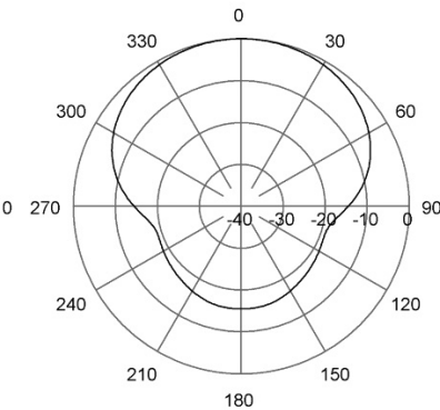
H-Plane | 123 MHz
