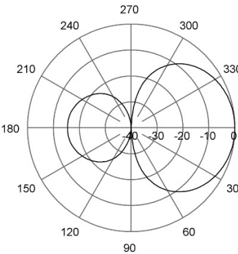
E-Plane | 123 MHz
