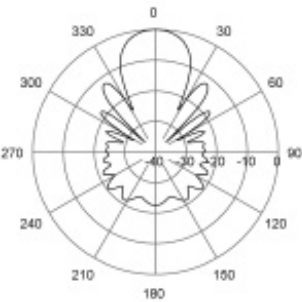
H-Plane | 788 MHz
