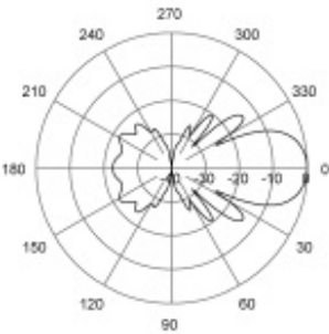
E-Plane | 788 MHz
