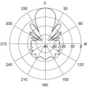
H-Plane | 497 MHz
