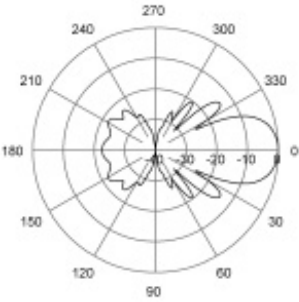
E-Plane | 497 MHz
