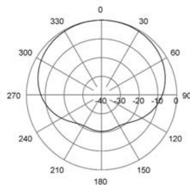
H-Plane | 104 MHz
