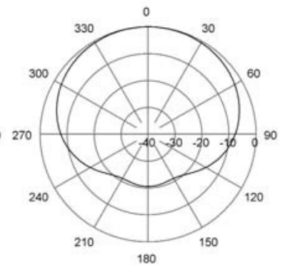
H-Plane | 85 MHz
