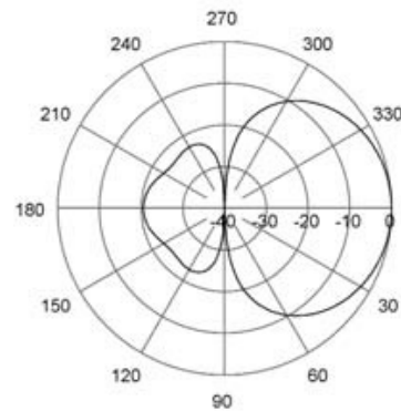
E-Plane | 85 MHz
