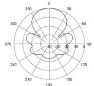
H-Plane | 455 MHz
