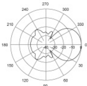
E-Plane | 410 MHz
