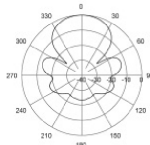
H-Plane | 410 MHz
