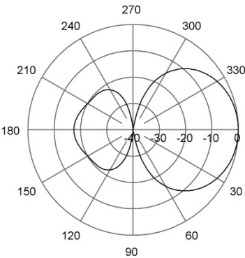
E-Plane | 455 MHz
