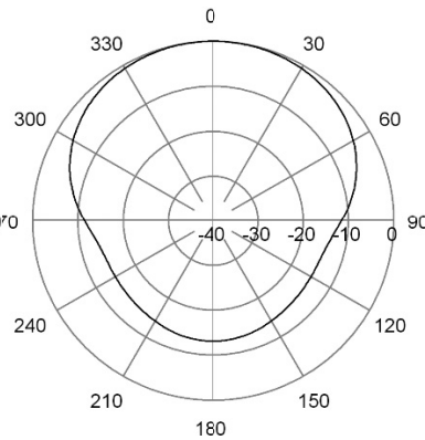
H-Plane | 185 MHz
