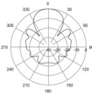
H-Plane | 460 MHz
