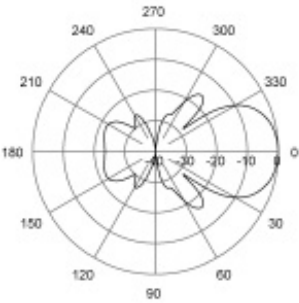
E-Plane | 460 MHz
