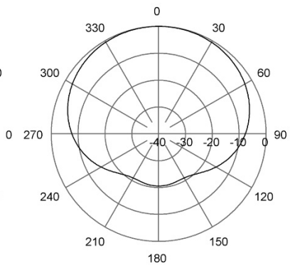
H-Plane | 165 MHz
