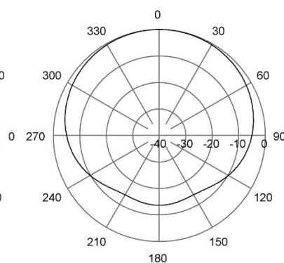
H-Plane | 50 MHz
