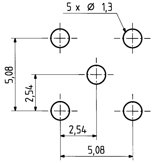
Montageloch ML 15
