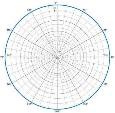
H-Plane | 875 MHz
