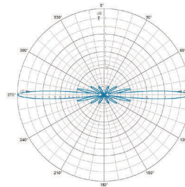
E-Plane | 780 MHz
