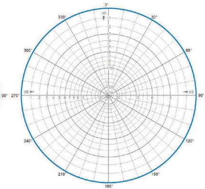
H-Plane | 875 MHz
