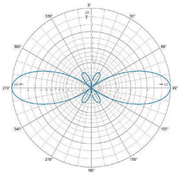
E-Plane | 445 MHz
