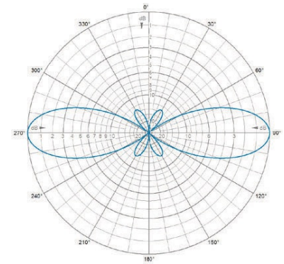
E-Plane | 420 MHz
