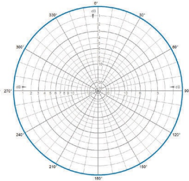
H-Plane | 132 MHz
