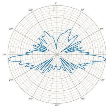
E-Plane | 875 MHz | 6°
