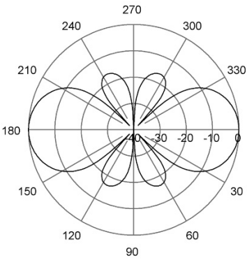
E-Plane | 200 MHz
