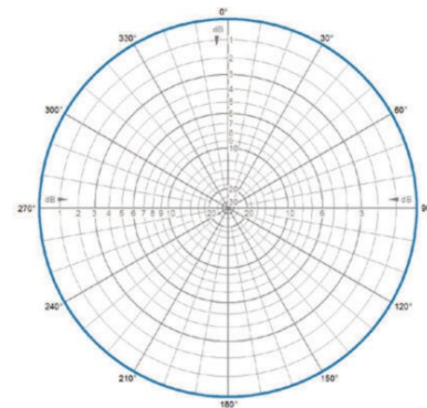
H-Plane | 445 MHz
