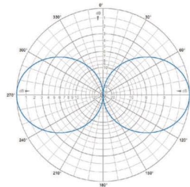
E-Plane | 445 MHz
