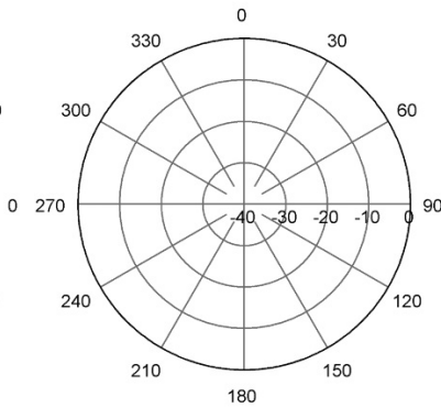
H-Plane | 155 MHz
