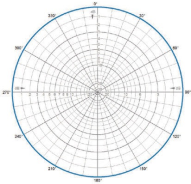
H-Plane | 184 MHz
