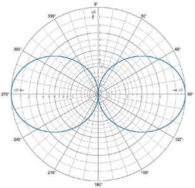
E-Plane | 184 MHz
