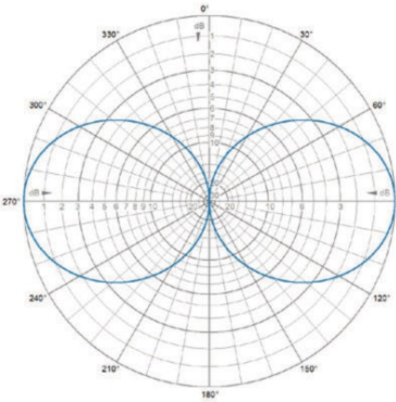
E-Plane | 250 MHz
