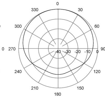
H-Plane | 144 MHz
