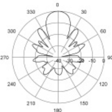
H-Plane | 396 MHz
