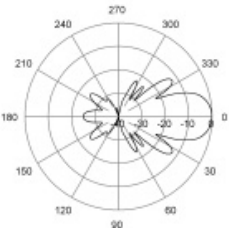
E-Plane | 396 MHz
