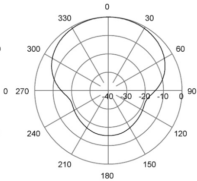
H-Plane | 102 MHz
