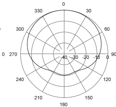
H-Plane | 184 MHz
