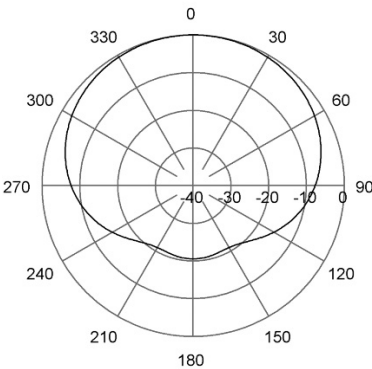
H-Plane | 455 MHz
