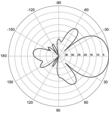
E-Plane | 1478 MHz
