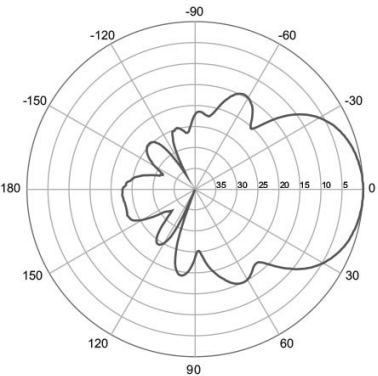
H-Plane | 1478 MHz
