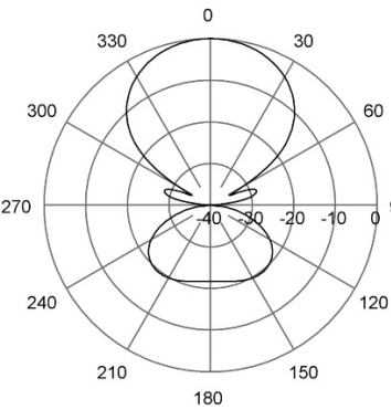
E-Plane | 146 MHz
