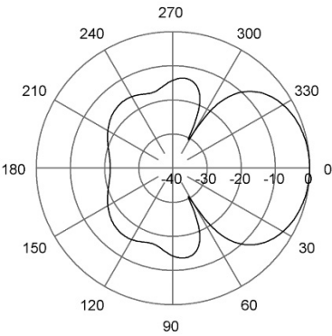
H-Plane | 146 MHz
