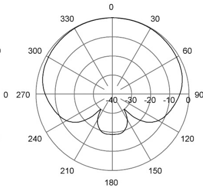
H-Plane | 460 MHz
