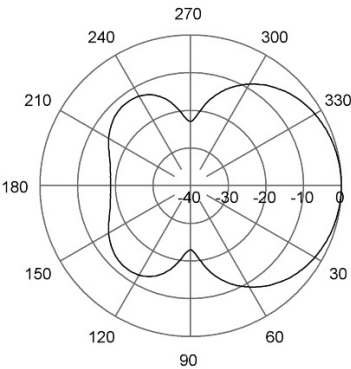
E-Plane | 460 MHz
