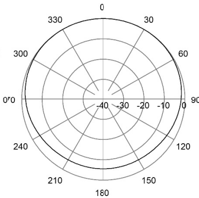
H-Plane | 162 MHz
