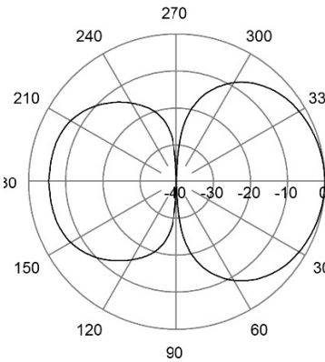
E-Plane | 162 MHz
