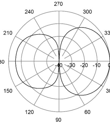
E-Plane | 158 MHz
