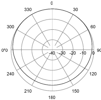
H-Plane | 158 MHz
