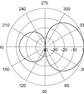
E-Plane | 185 MHz
