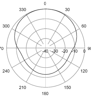
H-Plane | 78 MHz
