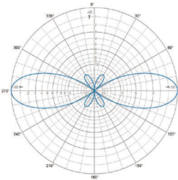
E-Plane | 222 MHz
