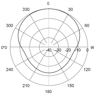
H-Plane | 165 MHz
