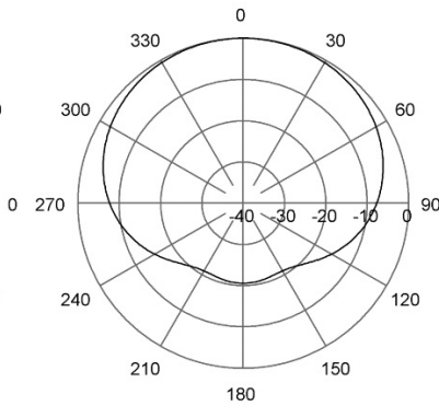
H-Plane | 154 MHz
