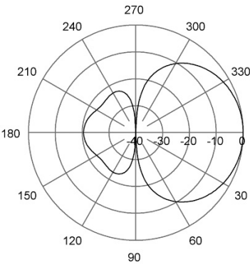
E-Plane | 154 MHz
