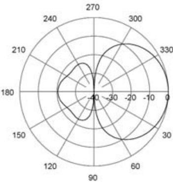
E-Plane | 220 MHz
