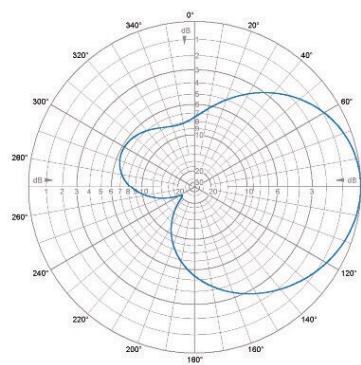
E-Plane | 425 MHz
