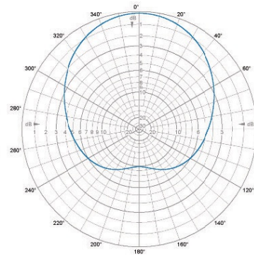
H-Plane | 425 MHz
