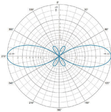
E-Plane | 312 MHz
