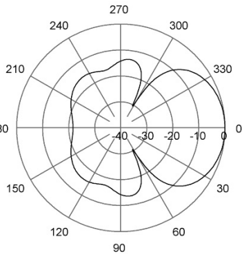
H-Plane | 420 MHz
