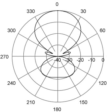
E-Plane | 420 MHz
