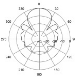
H-Plane | 460 MHz
