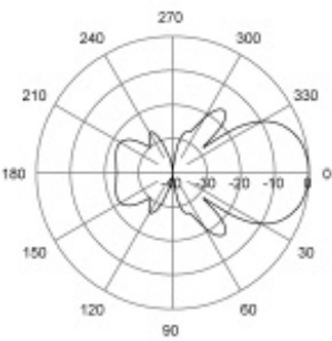
E-Plane | 460 MHz
