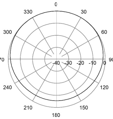
H-Plane | 98 MHz
