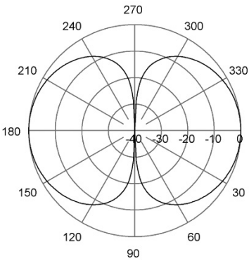
E-Plane | 185 MHz
