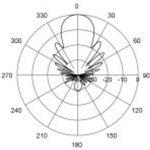
H-Plane | 1434 MHz
