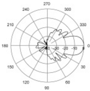
E-Plane | 1434 MHz
