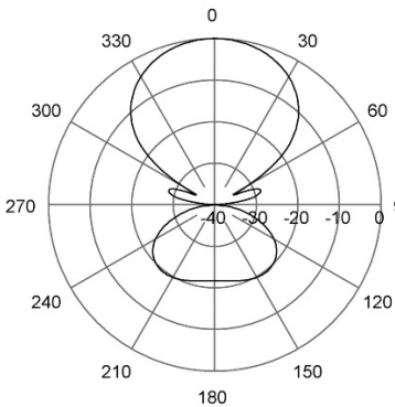
E-Plane | 428 MHz
