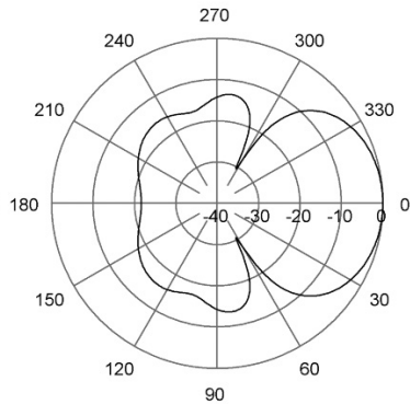
H-Plane | 428 MHz
